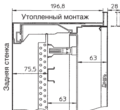
Панель с DIN-рейками
